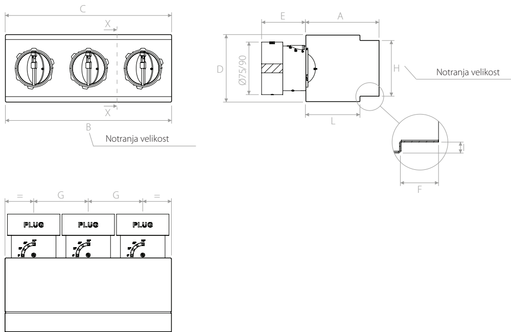
Prerez X-X
