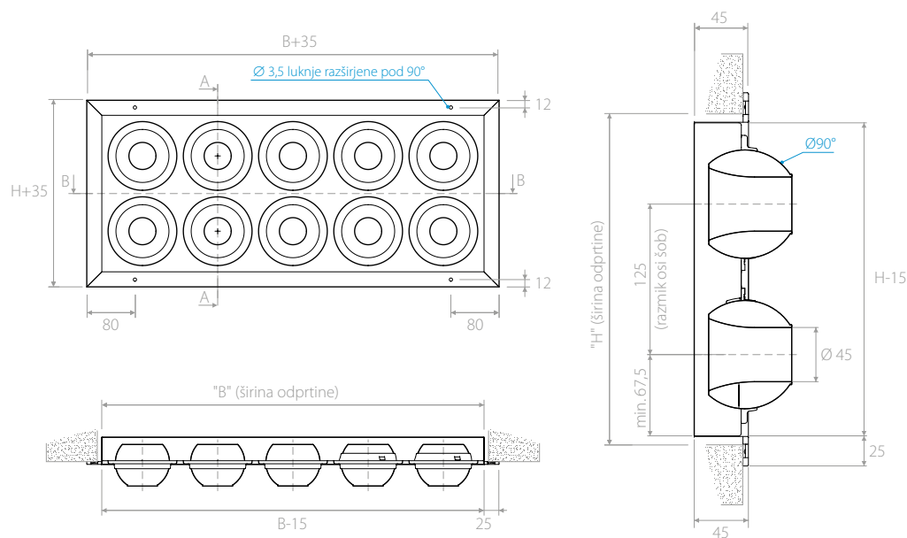
Prerez B-B
