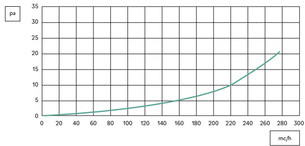
PLUGPVMCMR PERDITE DI CARICO PER SINGOLO FLUSSO | AIR PRESSURE DROP FOR SINGLE
